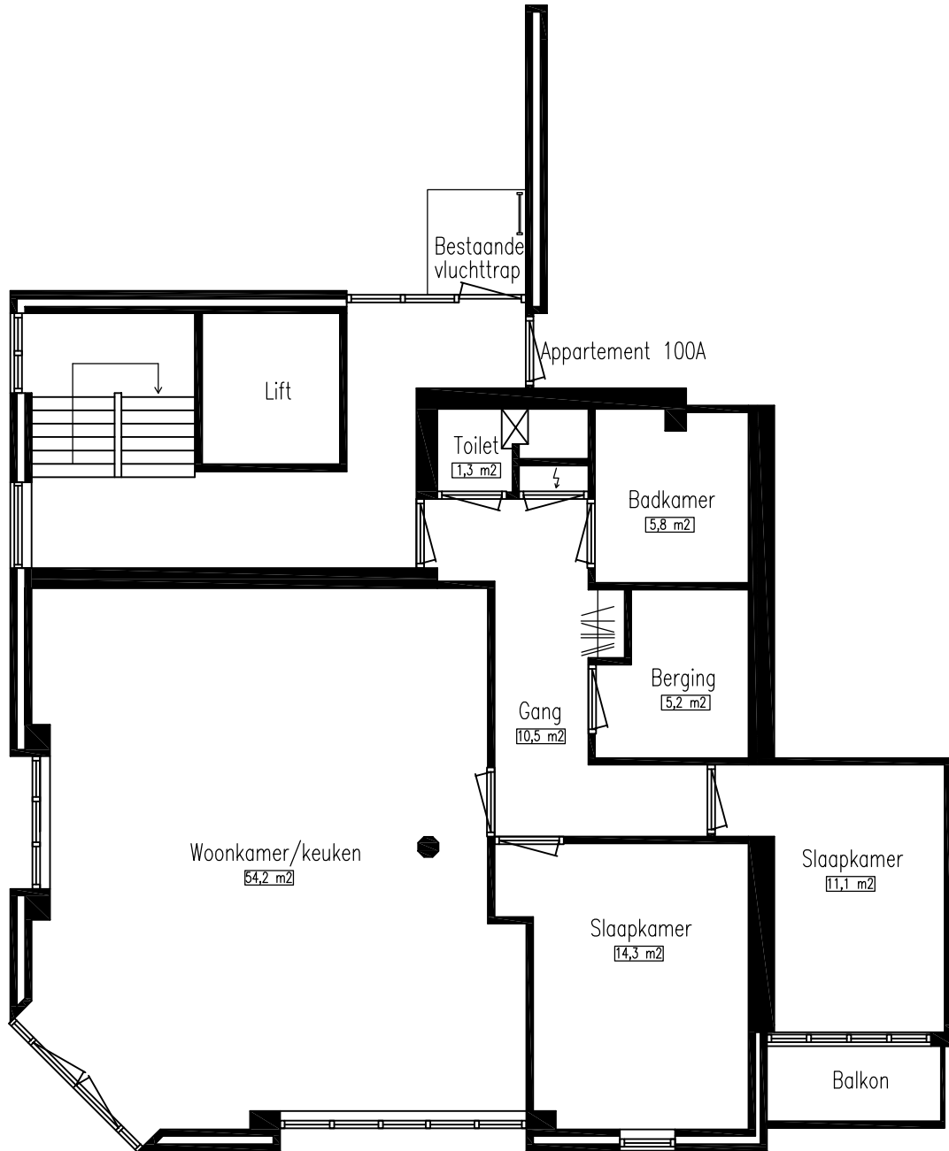
Plattegrond nieuw 1e verdieping appartement 100
